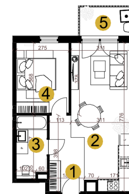
Rzut kondygnacji
