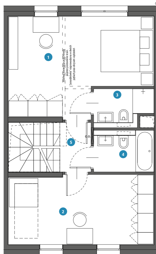
RZUT 1 PIĘTRA
