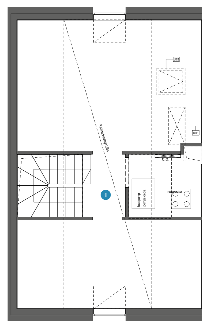
RZUT PODDASZA
