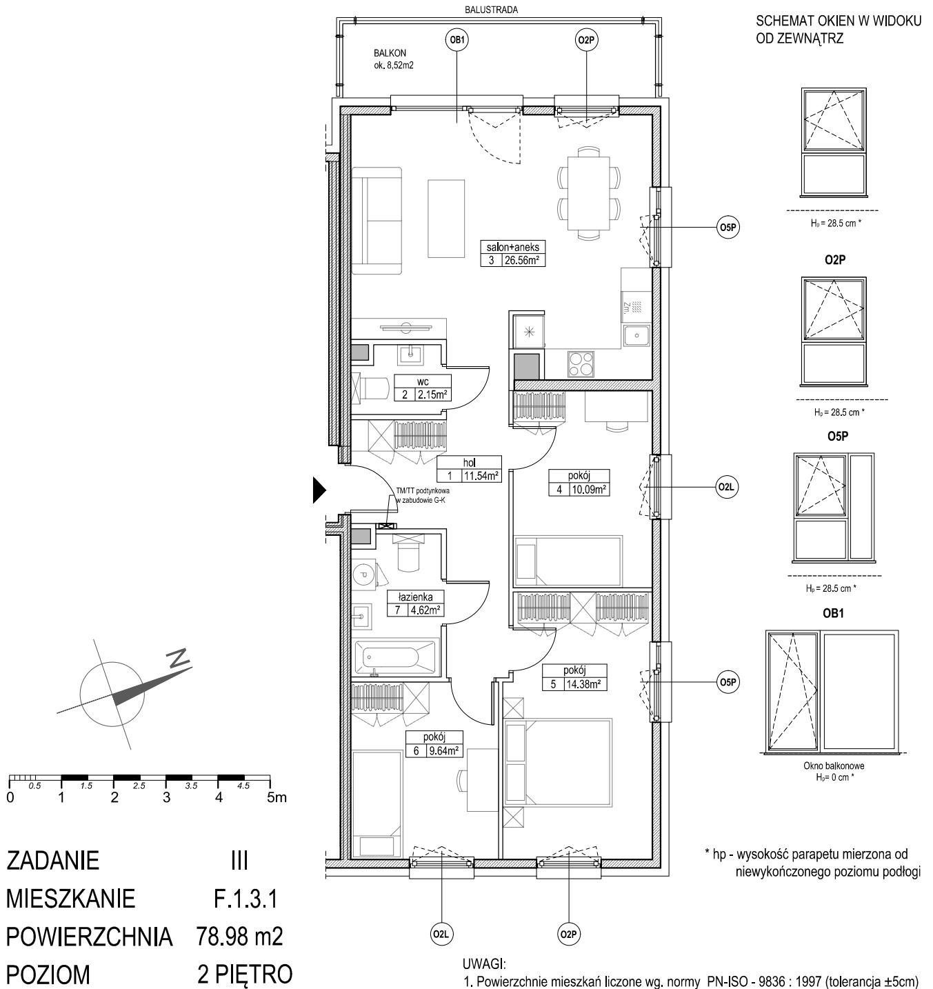
RZUT BUDYNKU F
