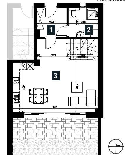
Rzut parteru
