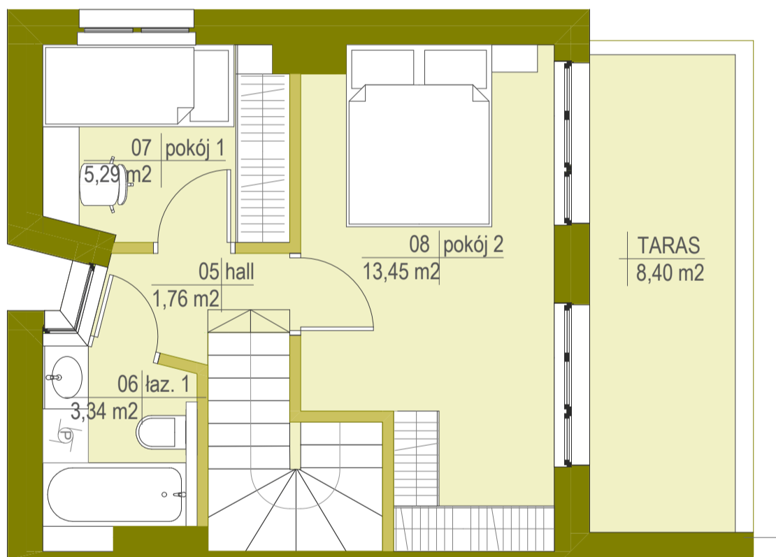
PIĘTRO I
