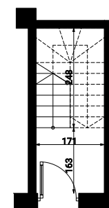
Rzut parteru
