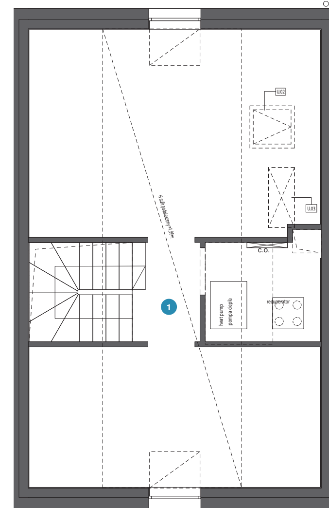
RZUT PODDASZA
