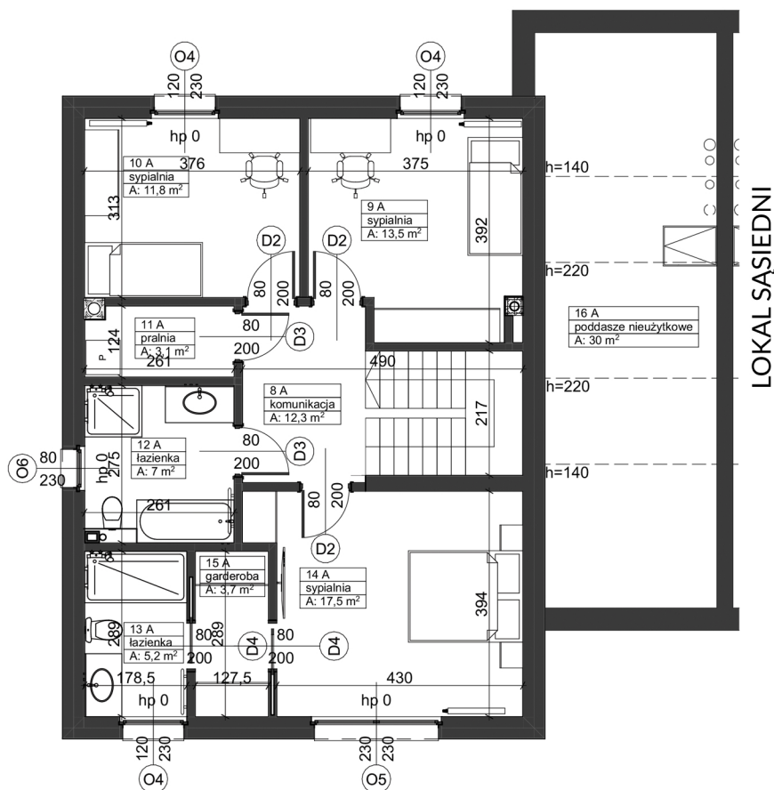
rzut piętra
