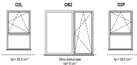
SCHEMAT OKIEN W WIDOKU OD ZEWNĄTRZ
