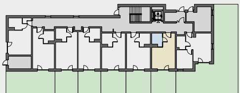
RZUT KONDYGNACJI
