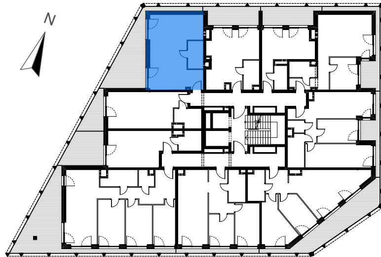
PIĘTRO 2 MIESZKANIE B.12
