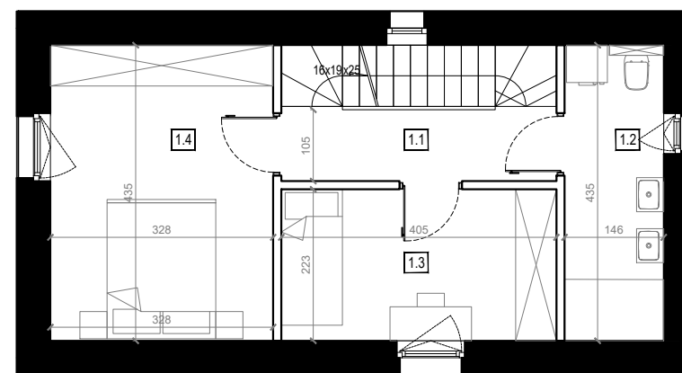
PIĘTRO I
