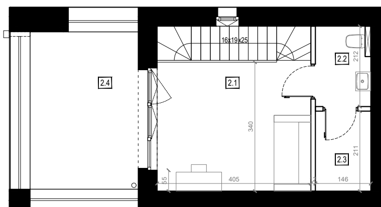
PIĘTRO II
