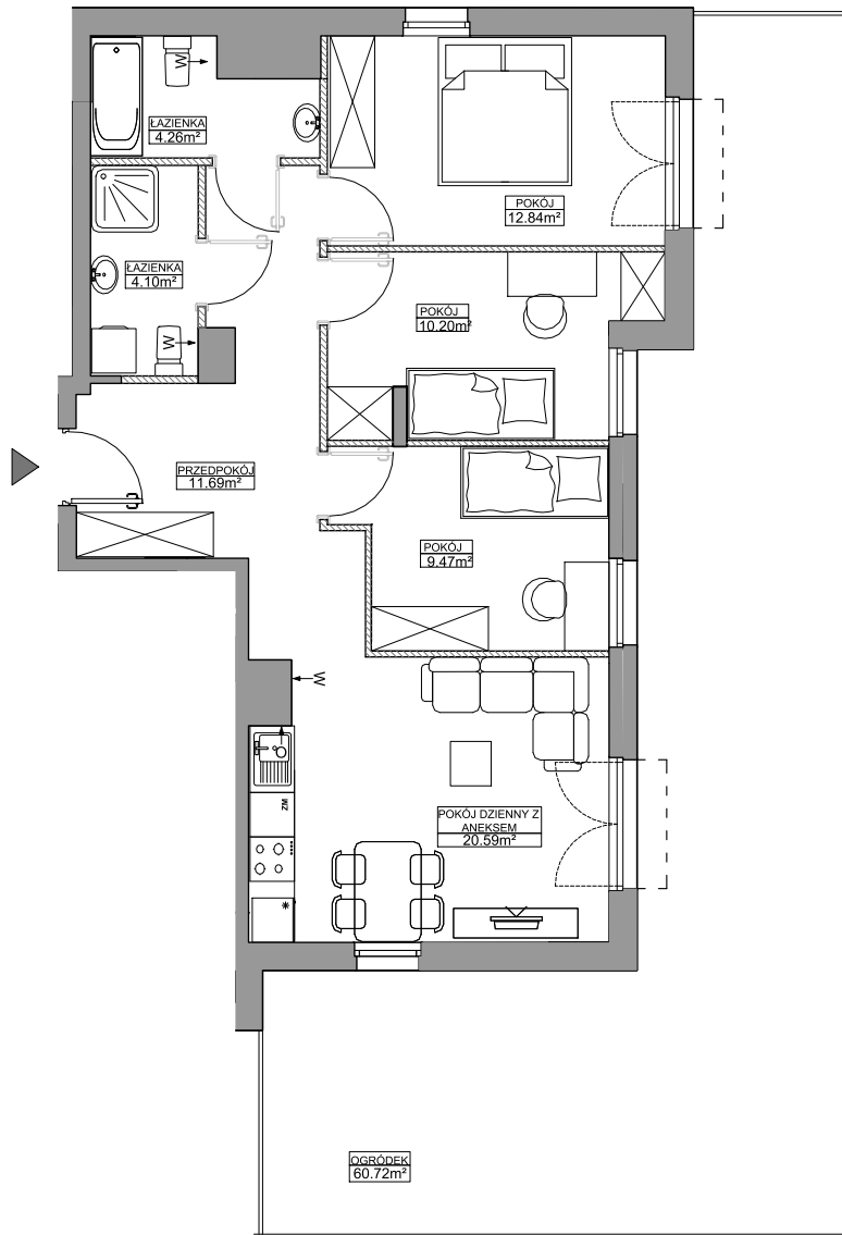
SCHEMAT LOKALU MIESZKALNEGO NA RZUCIE KONDYGNACJI
