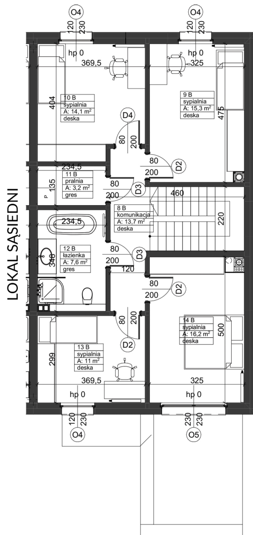
rzut piętra
