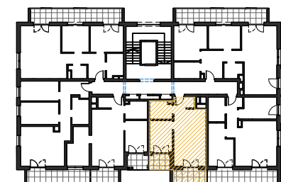
Schemat kondygnacji +3
