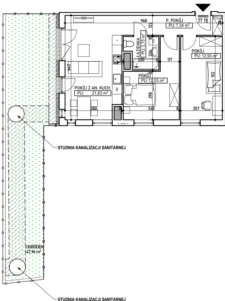
RZUT KONDYGNACJI PARTERU BUD. C Z ZAZNACZENIEM LOKALU MIESZKALNEGO
