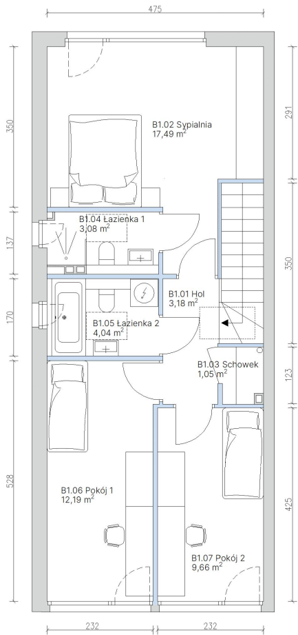
RZUT PIĘTRA
