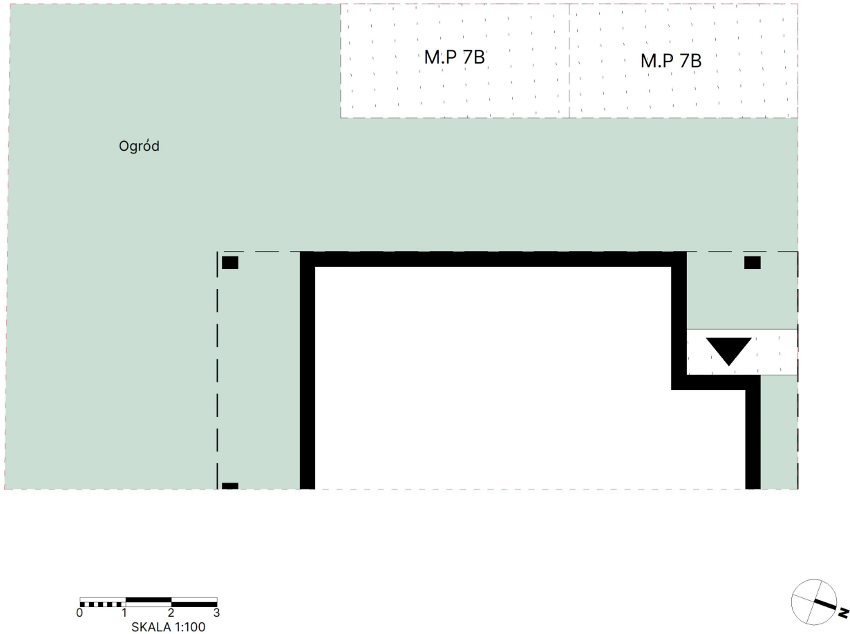
PLAN SYTUACYJNY
