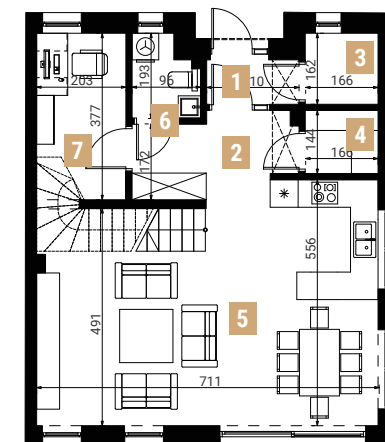
Rzut parteru
