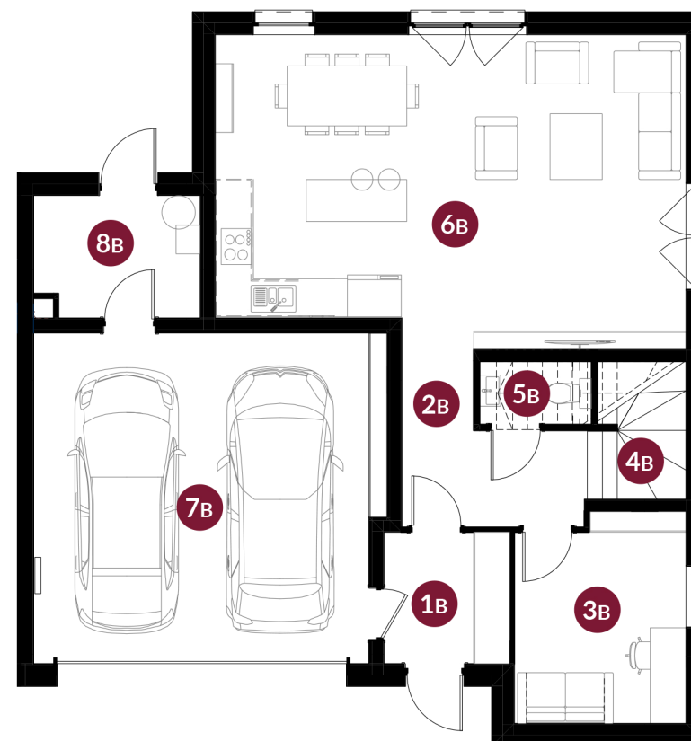
rzut parteru
