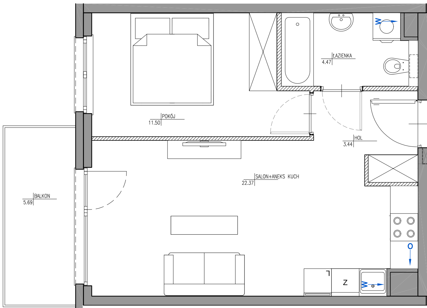
SCHEMAT LOKALU NA RZUCIE
