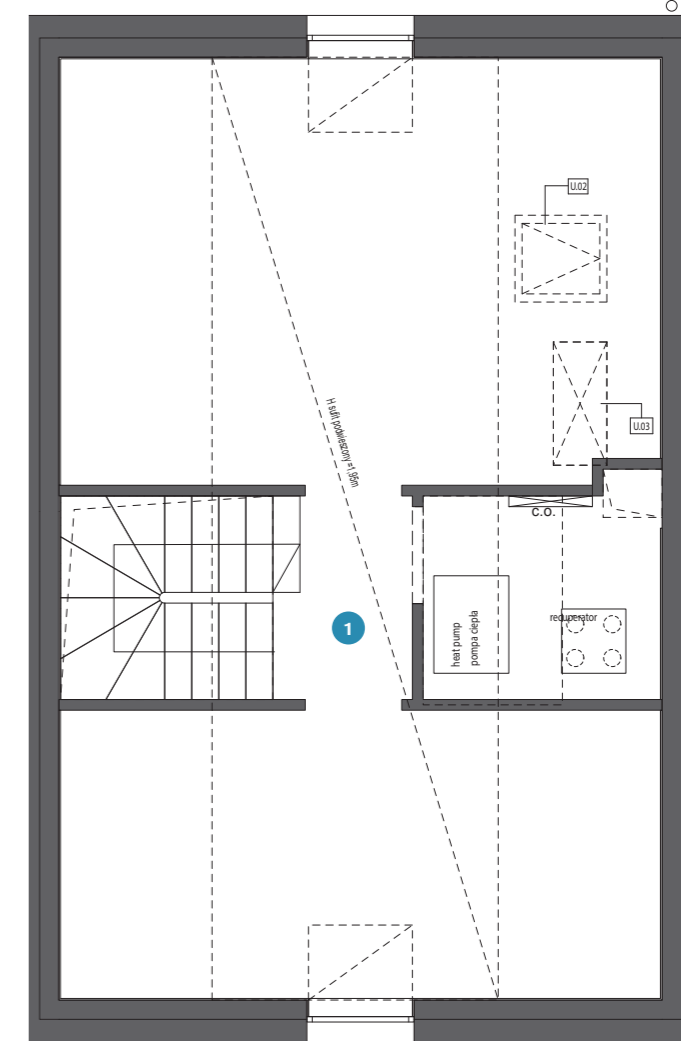
RZUT PODDASZA
