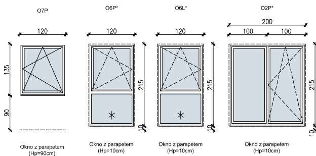
SCHEMAT OKIEN W WIDOKU OD WEWNĄTRZ:
