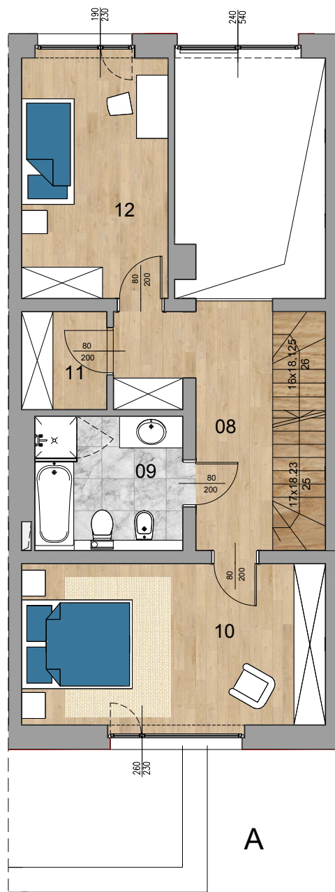
RZUT 1 PIETRA
