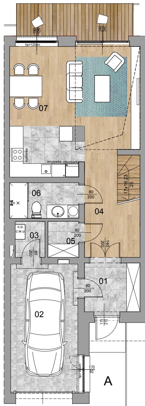
RZUT PARTERU
