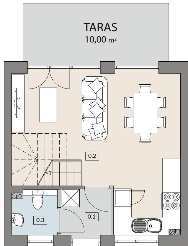
RZUT PARTERU
