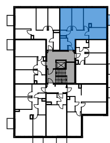
RZUT KONDYGNACJI 3 PIĘTRA BUD. A Z ZAZNACZENIEM LOKALU MIESZKALNEGO
