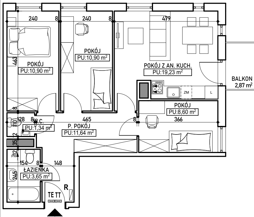
RZUT KONDYGNACJI 3 PIĘTRA BUD. A Z ZAZNACZENIEM LOKALU MIESZKALNEGO
