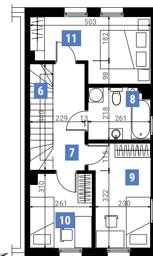
Rzut piętra
