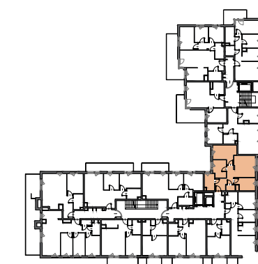
SCHEMAT KONDYGNACJI
