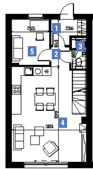
Rzut parteru
