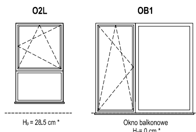
SCHEMAT OKIEN W WIDOKU OD ZEWNĄTRZ
