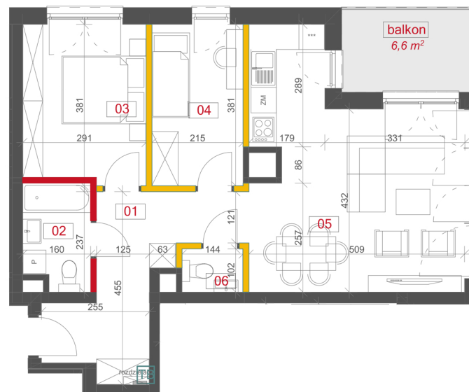
BUDYNEK B
