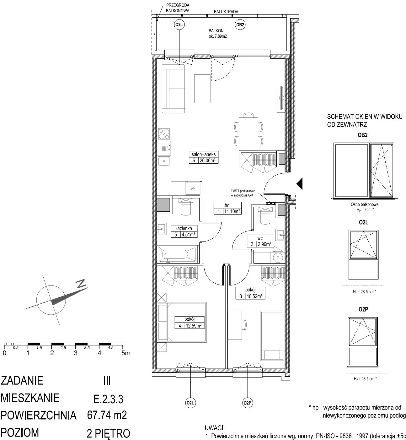
RZUT BUDYNKU E
