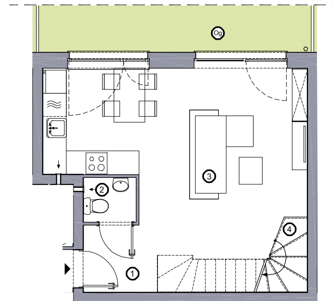
Rzut parteru
