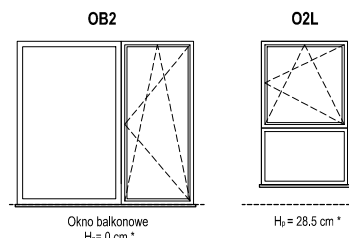
SCHEMAT OKIEN W WIDOKU OD ZEWNĄTRZ
