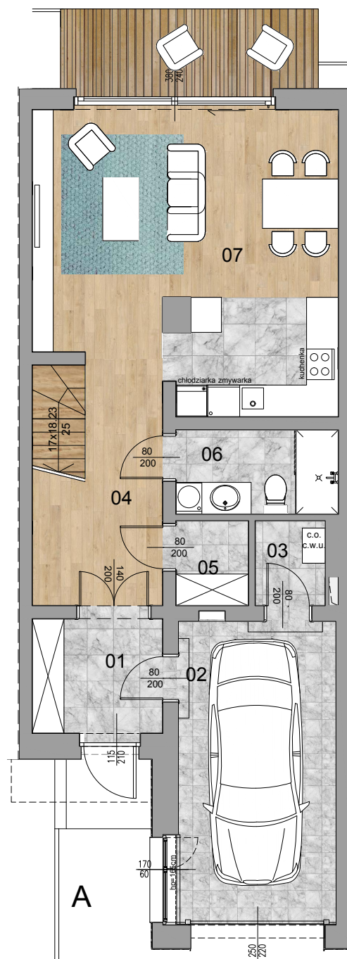
RZUT PARTERU
