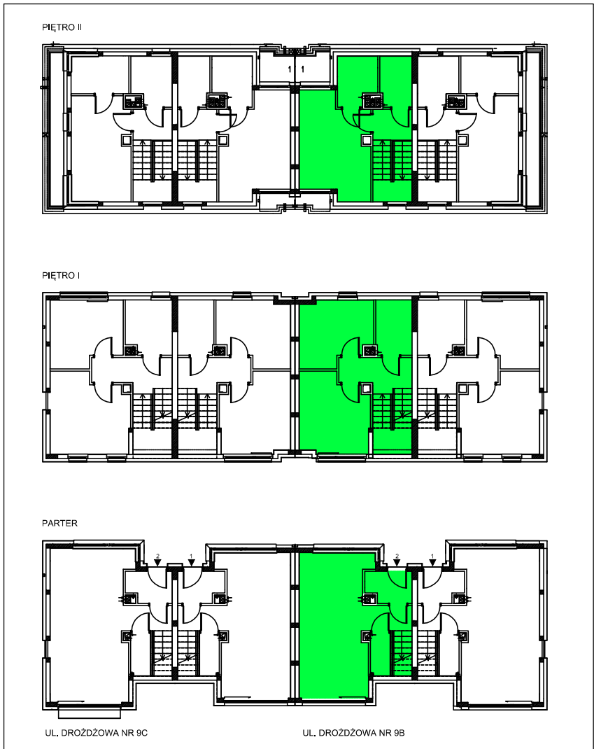
SCHEMAT KONDYGNACJI BUDYNKU NR 9B, 9C.
