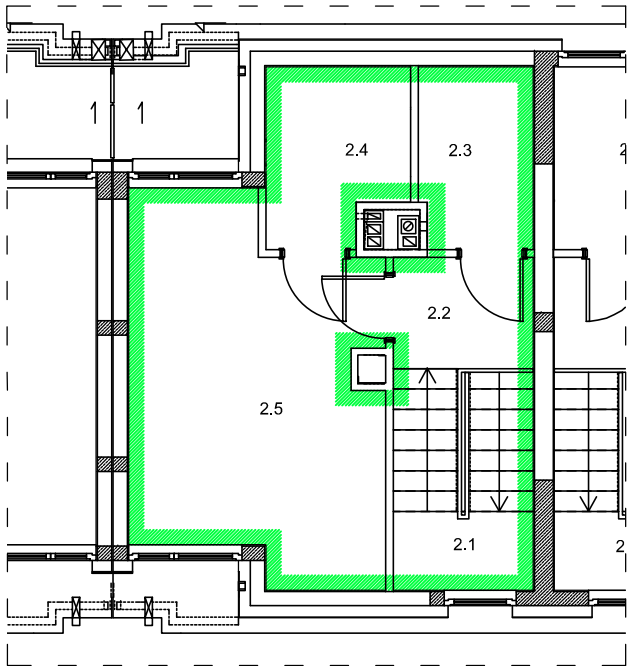
RZUT PIĘTRA II-GO BUDYNKU NR 9B LOKAL MIESZKALNY NR 2
