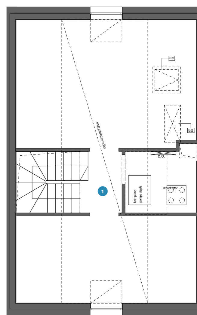
RZUT PODDASZA
