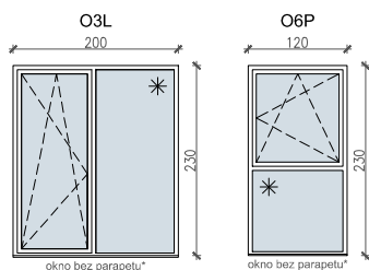
SCHEMAT OKIEN W WIDOKU OD WEWNĄTRZ:
