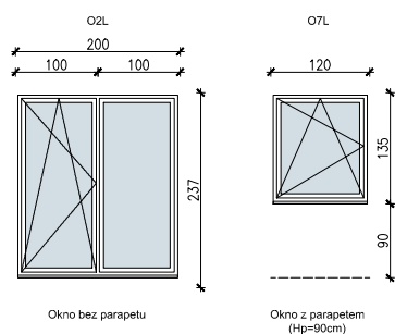
SCHEMAT OKIEN W WIDOKU OD WEWNĄTRZ:
