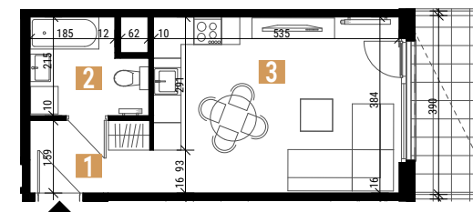
Rzut mieszkania
