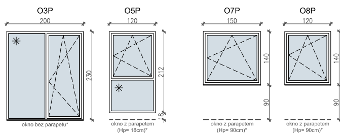
SCHEMAT OKIEN W WIDOKU OD WEWNĄTRZ:
