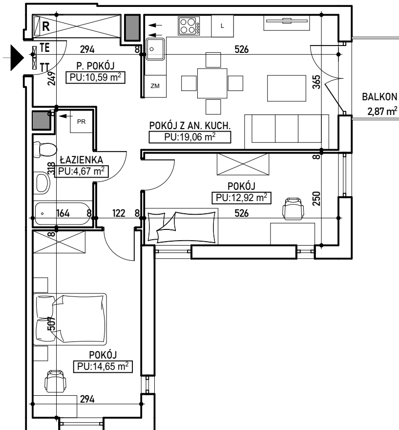
RZUT KONDYGNACJI 3 PIĘTRA BUD. A Z ZAZNACZENIEM LOKALU MIESZKALNEGO
