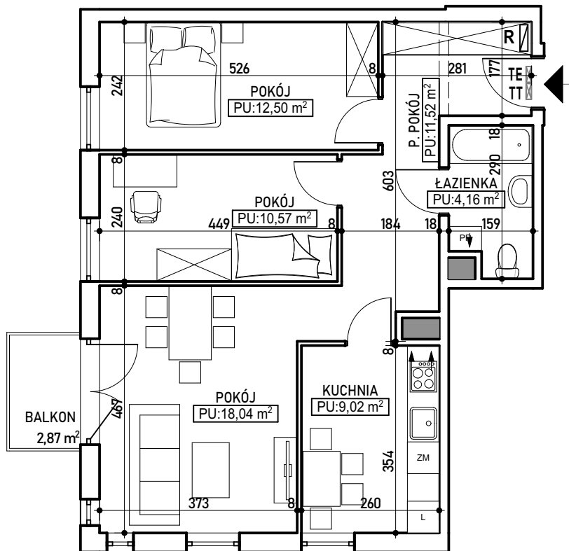
RZUT KONDYGNACJI 2 PIĘTRA BUD. C Z ZAZNACZENIEM LOKALU MIESZKALNEGO
