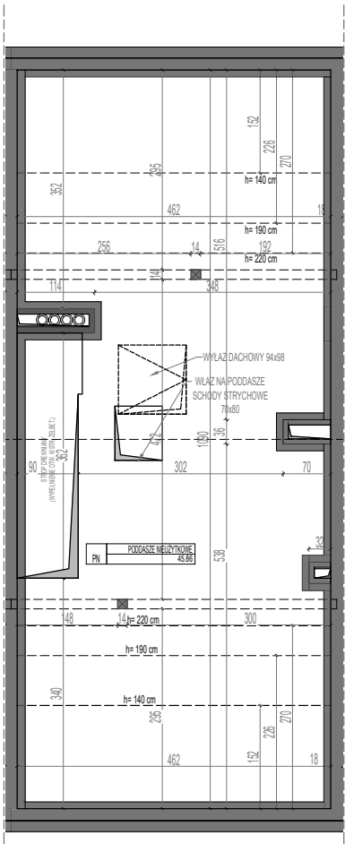
PODDASZE
