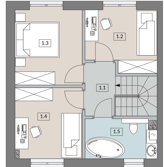
RZUT PIĘTRA
