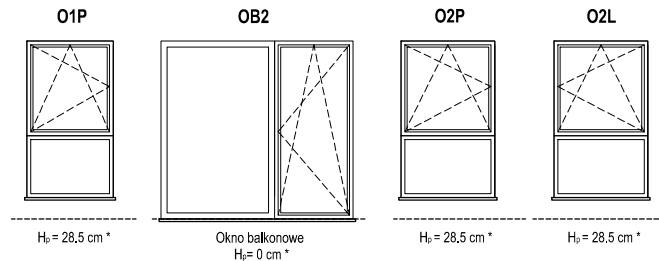
SCHEMAT OKIEN W WIDOKU OD ZEWNĄTRZ
