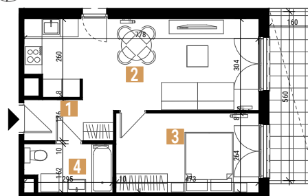
Rzut mieszkania
