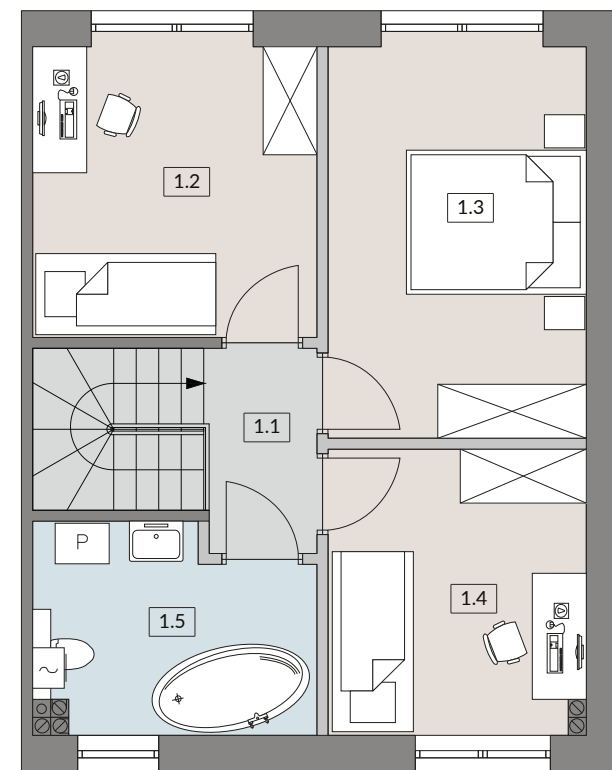
RZUT PIĘTRA
