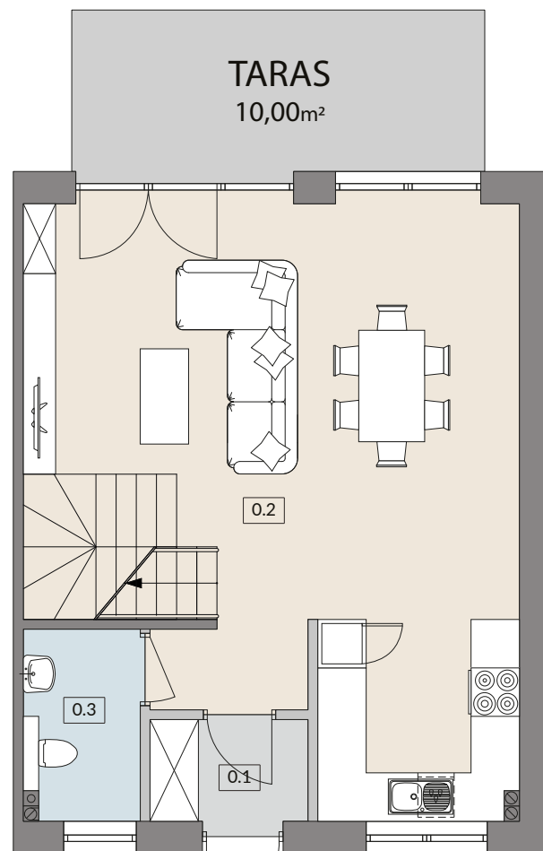
RZUT PARTERU
