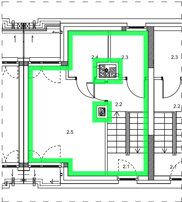
RZUT PIĘTRA II-GO BUDYNKU NR 11K LOKAL MIESZKALNY NR 2
