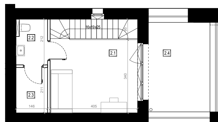
PIĘTRO II
