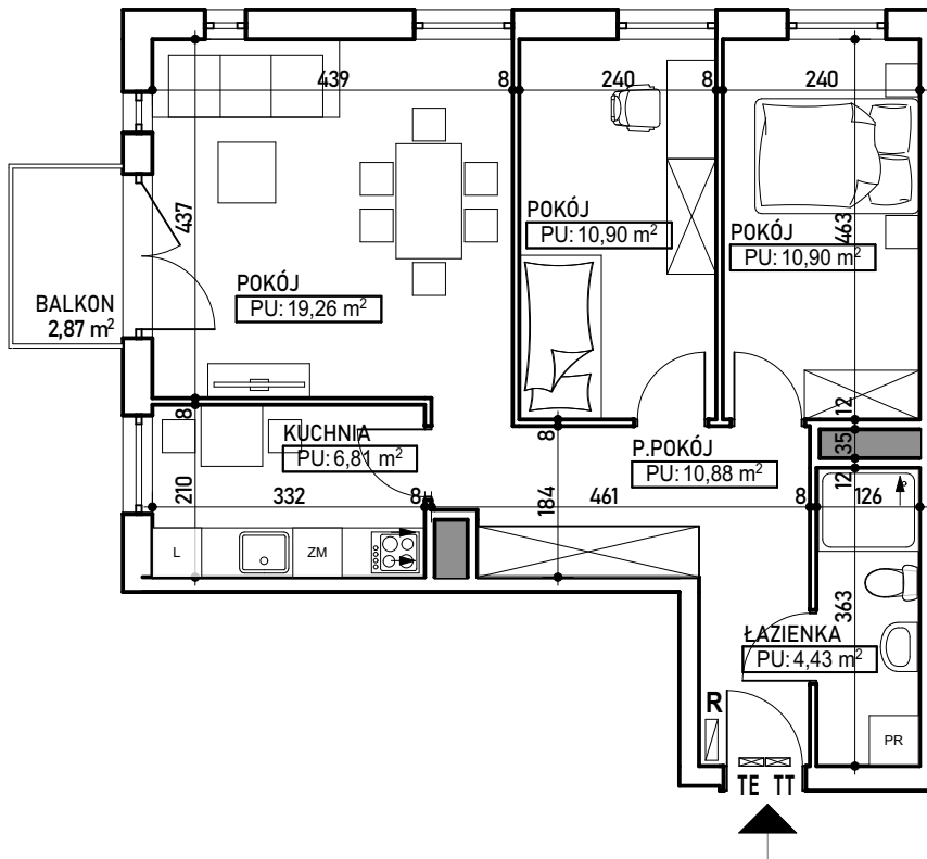
RZUT KONDYGNACJI 1 PIĘTRA BUD. A Z ZAZNACZENIEM LOKALU MIESZKALNEGO
